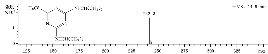
图 B.5 扑草净的质谱图
